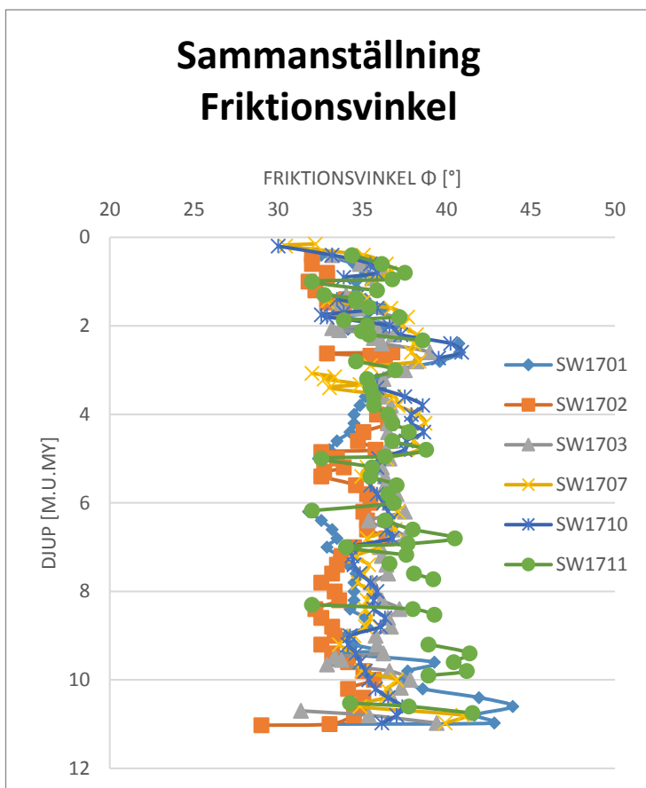
Figur 3: Sammanställning av friktionsvinkel.
