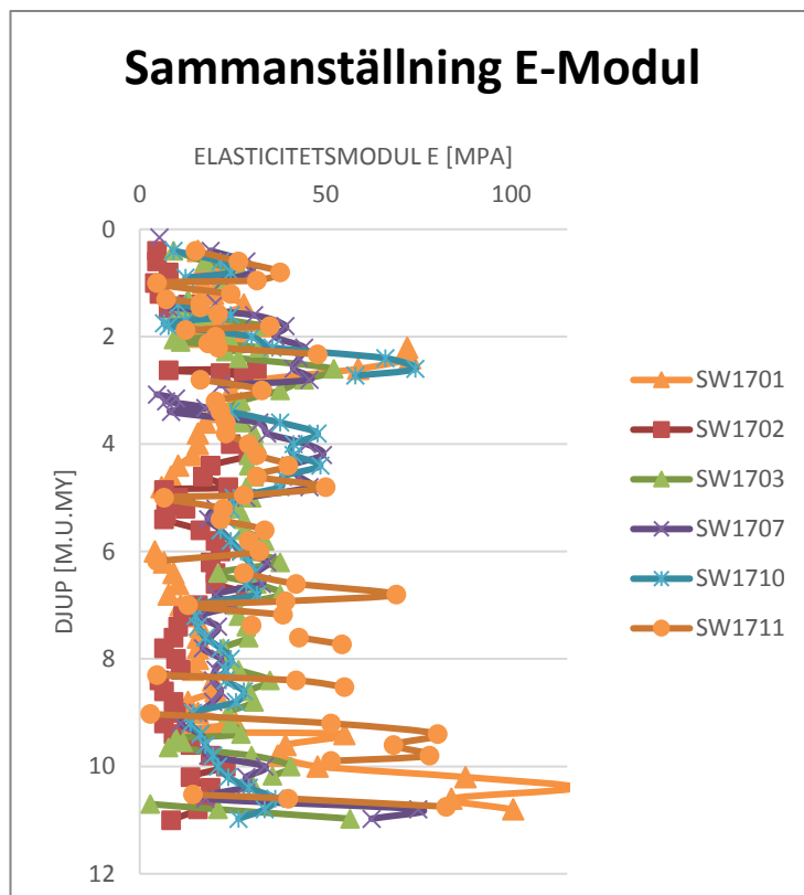
Figur 2: Sammanställning av E-modul.
